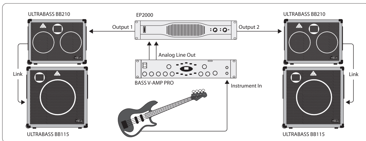
Bild 3.4: Utvidgad stereo-installation
