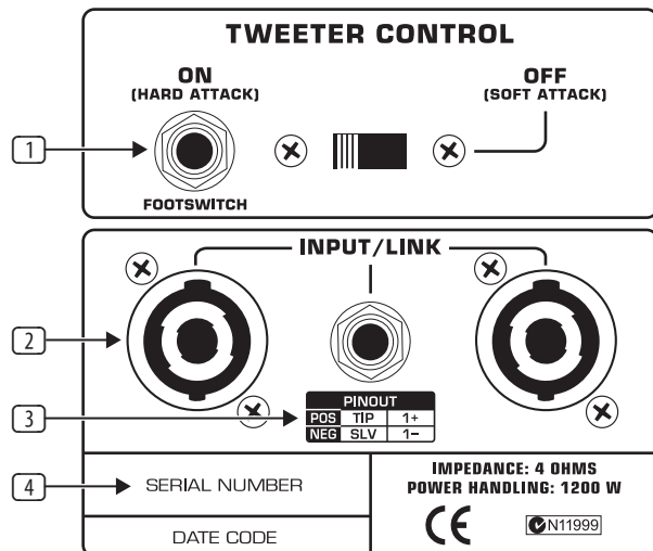
Bild 2.1: Reglage och anslutningar
