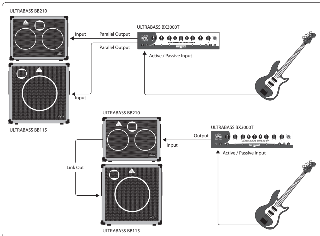
Bild 3.2: Utvidgad mono-installation med olika anslutningsmöjligheter för högtalarna
