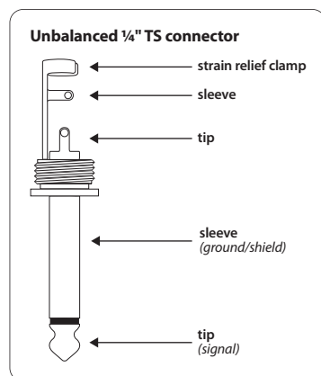
Bild 4.3: 6,3-mm monokontakt
