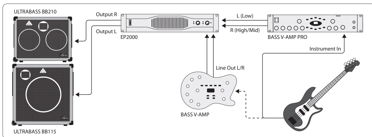
Bild 3.3: Bi-amping: basfrekvenser och diskanter återges fördelat via baslådorna
