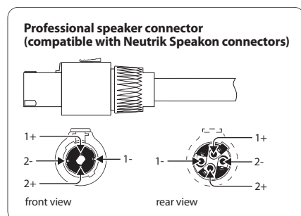
Bild 4.2: Professionell högtalaranslutning med polerna
