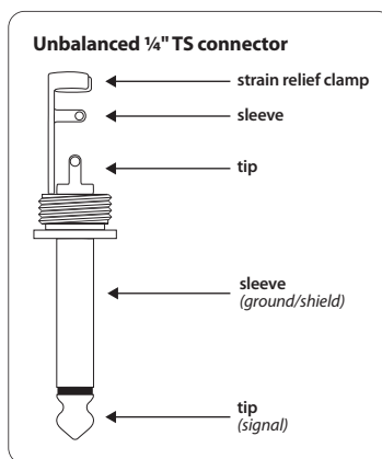
Fig. 4.3: presa jack 6,3 mm mono
