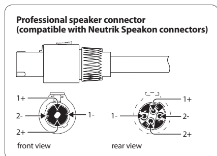
Fig. 4.2: collegamento degli altoparlanti per uso professionale con la polarità
