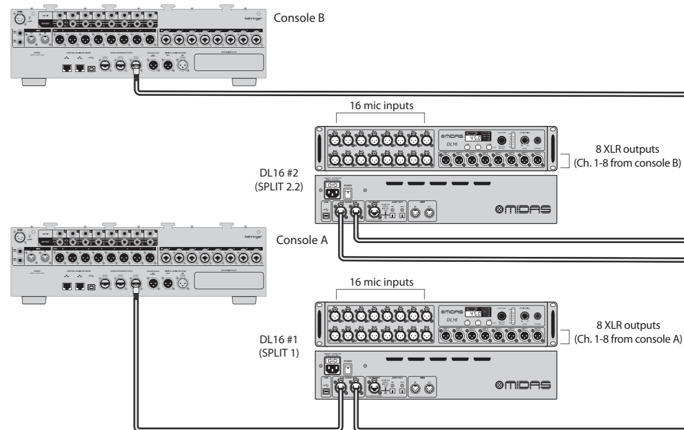
Fig. 5: Configuração de duas unidades com duas consolas e DL16s nos modos Split 1.3 e Split 2.2
