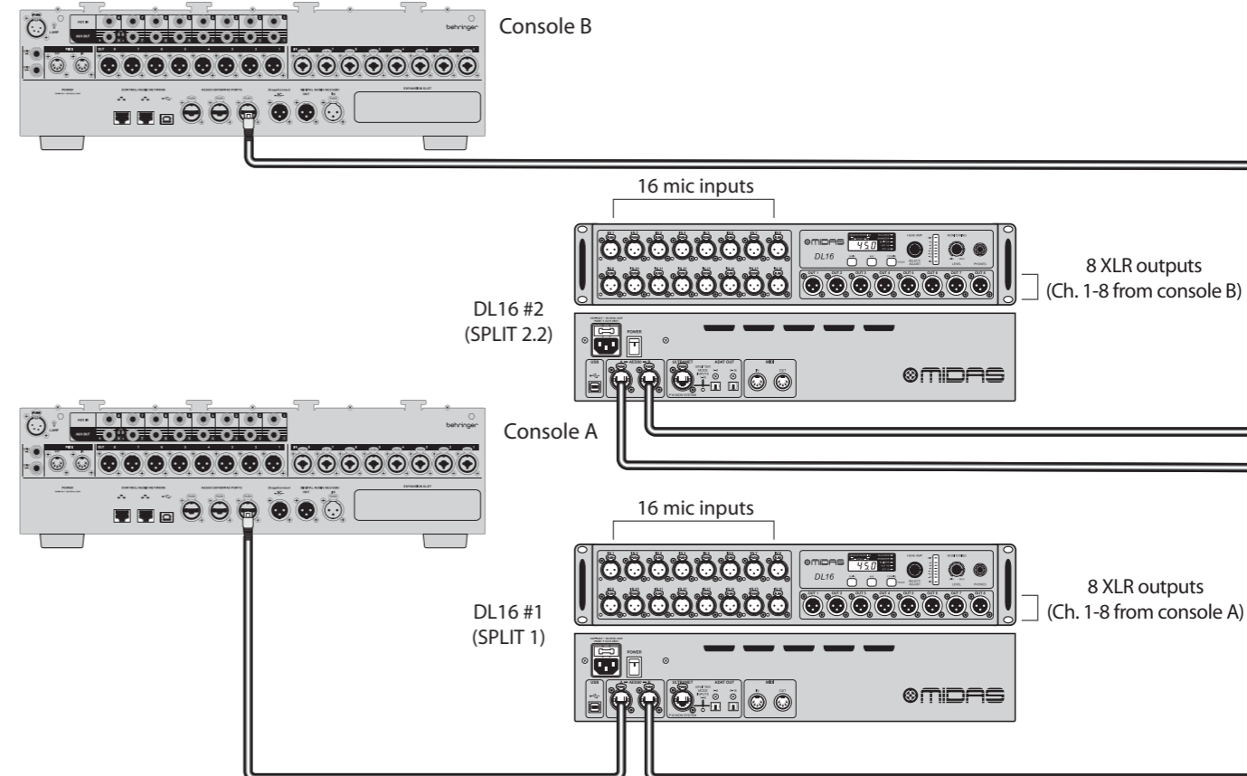
Fig. 5: Opstelling met twee eenheden met twee consoles en DL16's in Split 1.3 en Split 2.2 modi
