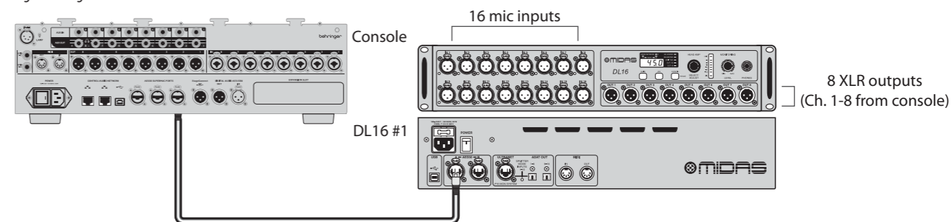
Fig. 1: Configuration d'une seule unité avec DL16 en mode Standard
