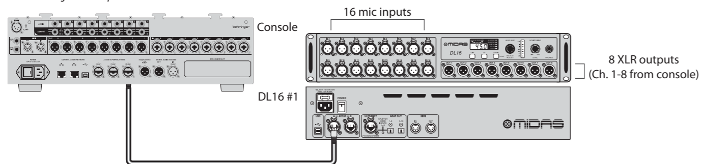
Abb. 1: Einzelgeräte-Setup mit DL16 im Standardmodus
