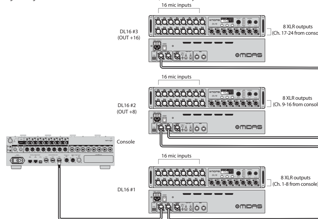
Fig. 2: Configuración de tres unidades con DL16s en modo Estándar, Estándar +8 y Estándar +16
