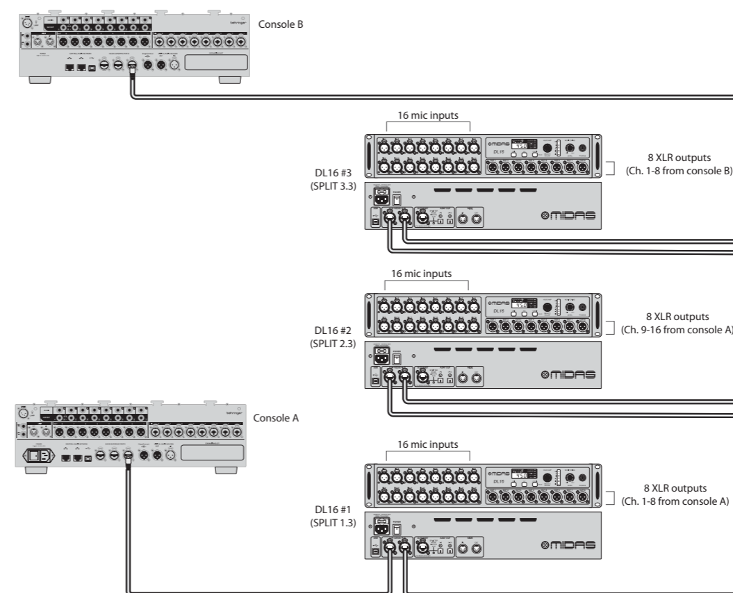
Fig. 4: Configuración de tres unidades con dos consolas y DL16s en modos Split 1.3, Split 2.3 y Split 3.3
