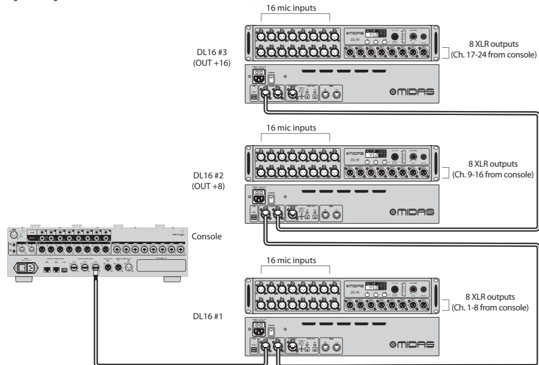
Fig. 2: Configuration de trois unités avec DL16 en mode Standard, Standard +8 et Standard +16
