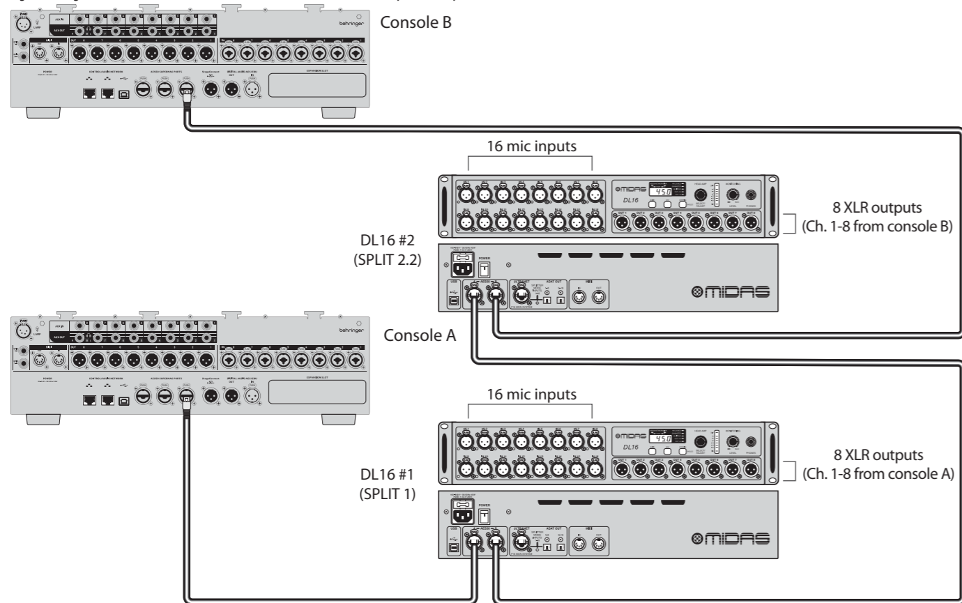
Fig. 5: Configurazione a due unità con due console e DL16 in modalità Split 1.3 e Split 2.2
