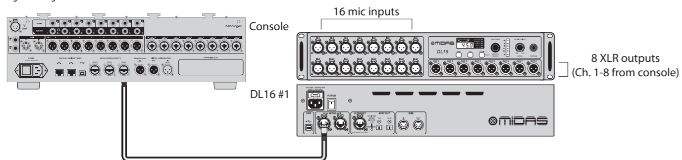
Fig. 1: Configuración de una sola unidad con DL16 en modo Estándar
