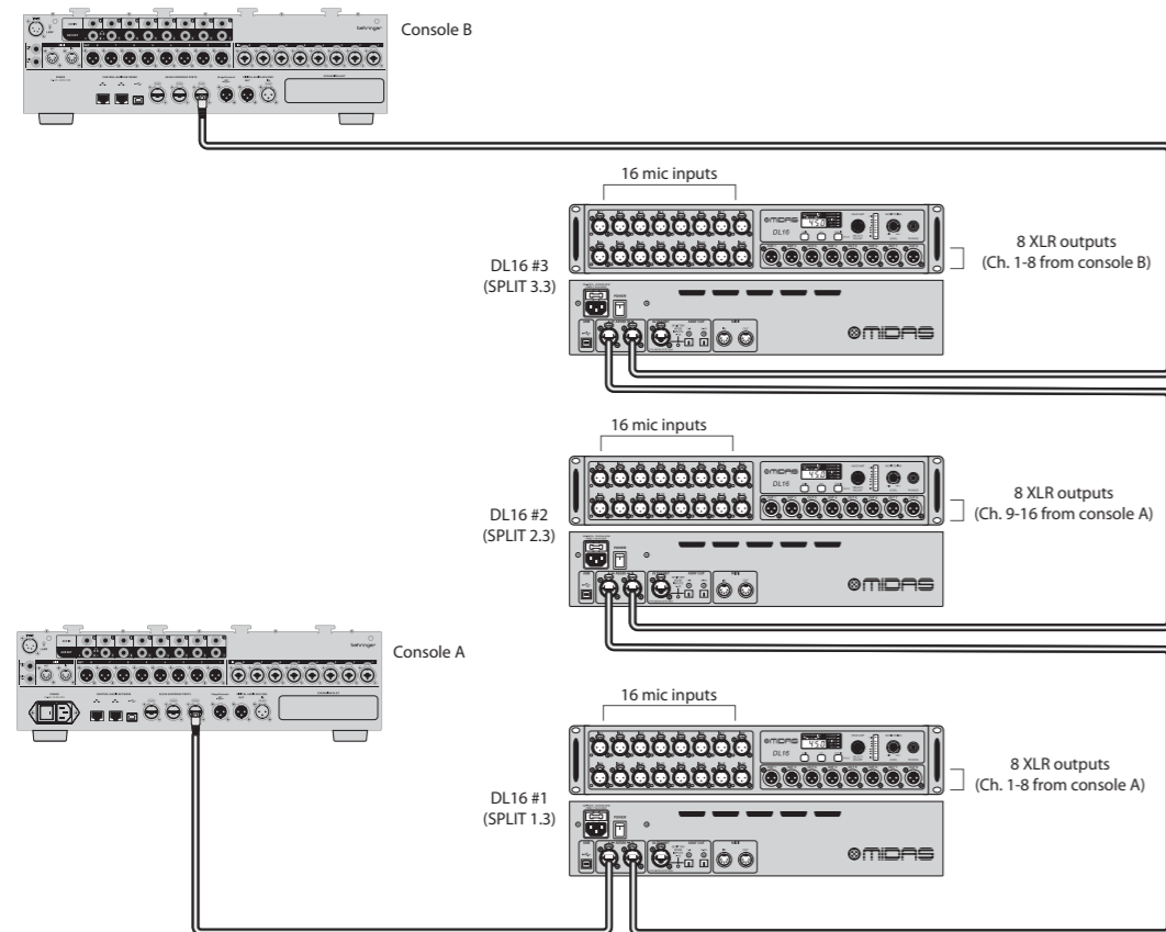
图 4: Split 1.3, Split 2.3 和 Split 3.3 模式的 DL16s 与两台控制台的三单元设置
