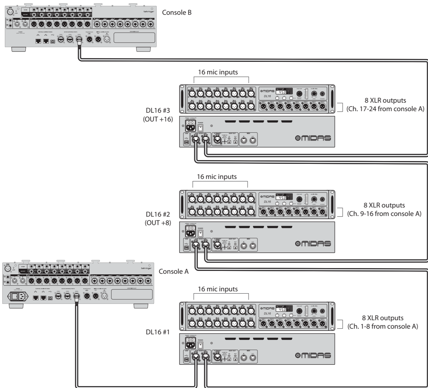
Abb. 3: Drei-Geräte-Setup mit zwei Konsolen und DL16s im Standardmodus, Standard +8 und Standard +16
