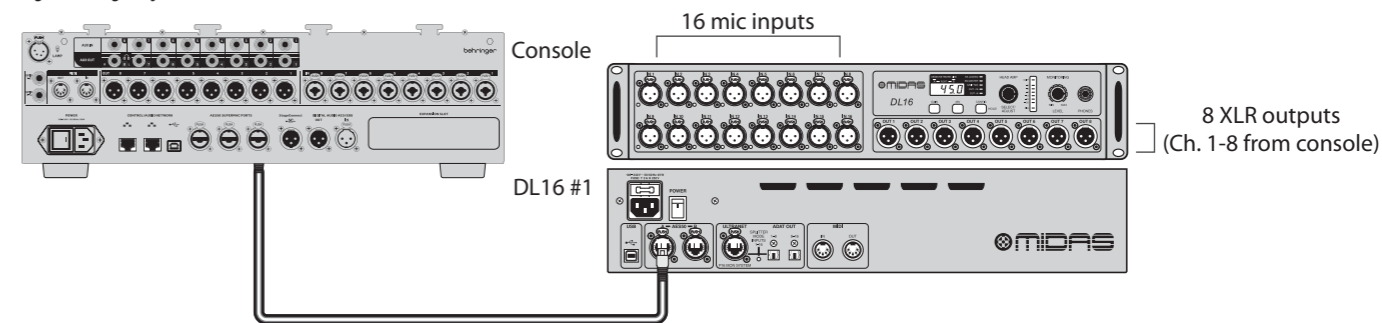
Fig. 1: Configuração de uma única unidade com DL16 no modo Padrão
