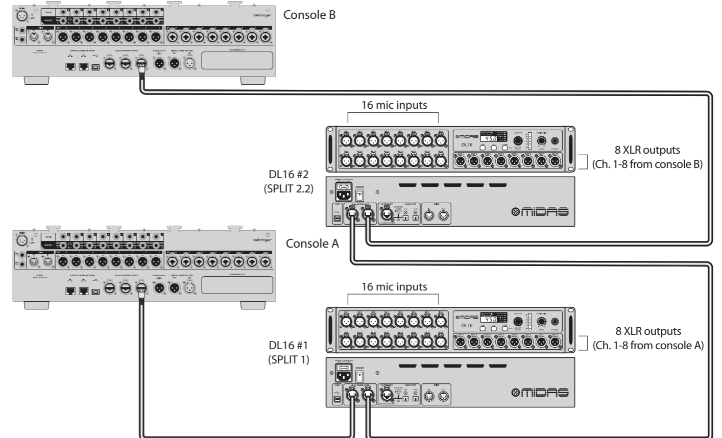
Fig. 5: Configuration à deux unités avec deux consoles et DL16s en modes Split 1.3 et Split 2.2
