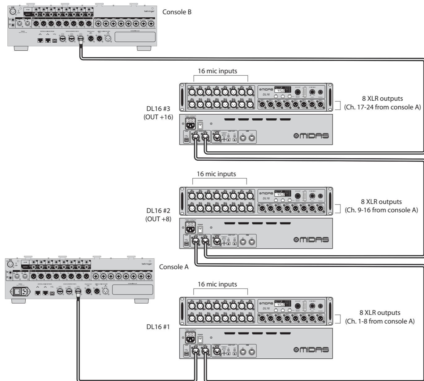
Fig. 3: Configuración de tres unidades con dos consolas y DL16s en modo Estándar, Estándar +8 y Estándar +16
