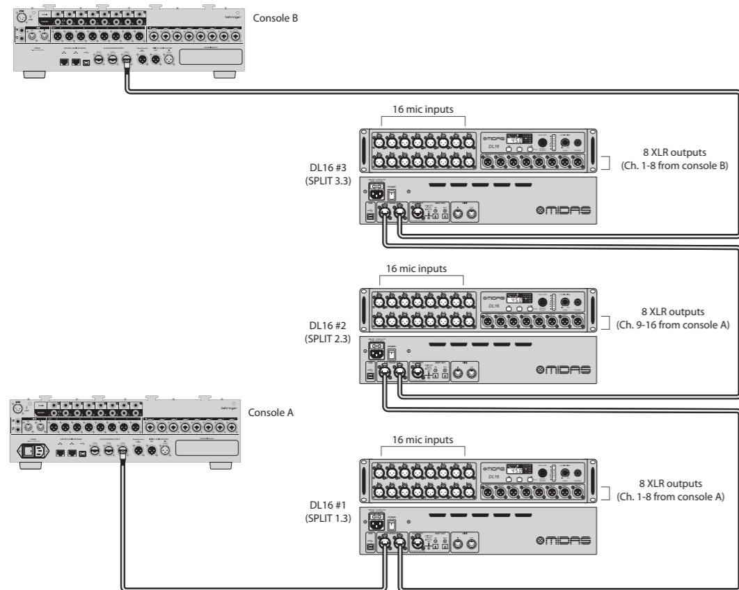
Rys. 4: Ustawienie trzech jednostek z dwoma konsolami i DL16 w trybach Split 1.3, Split 2.3 i Split 3.3
