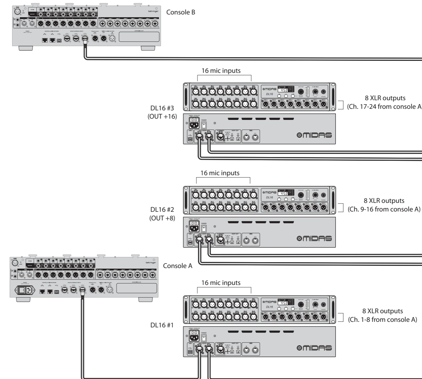
Fig. 3: Opstelling met drie eenheden met twee consoles en DL16's in Standaard modus, Standaard +8 en Standaard +16
