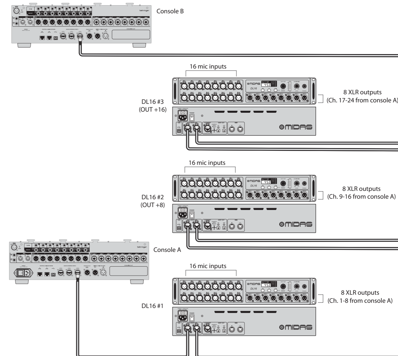
Rys. 3: Konfiguracja trzech jednostek z dwoma konsolami i DL16 w trybie Standard, Standard +8 i Standard +16
