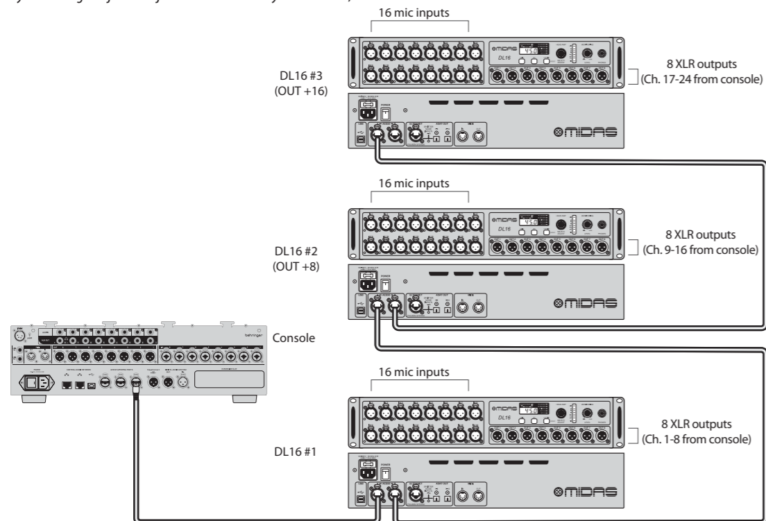
Rys. 2: Konfiguracja trzech jednostek z DL16 w trybie Standard, Standard +8 i Standard +16
