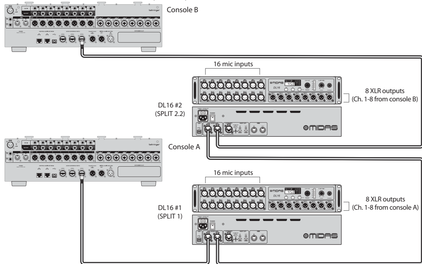
Abb. 5: Zwei Geräte in Reihe mit zwei Konsolen und DL16s im Split 1.3 und Split 2.2 Modus
