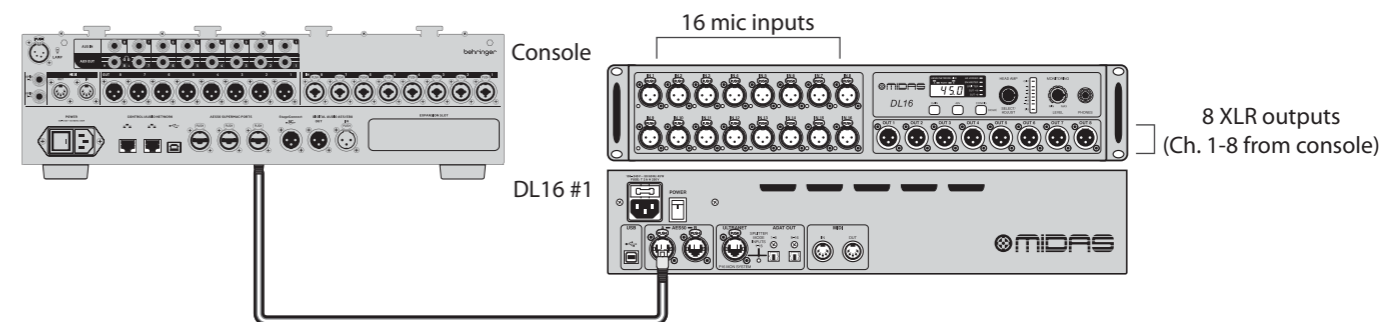
图 1: Standard 模式的 DL16 单元设置
