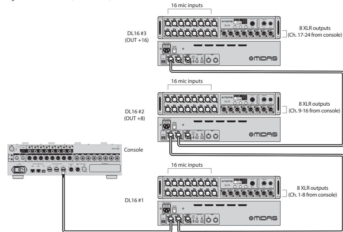
Fig. 2: Standard モード、Standard +8、および Standard +16 の DL16 での 3 ユニットのセットアップ
