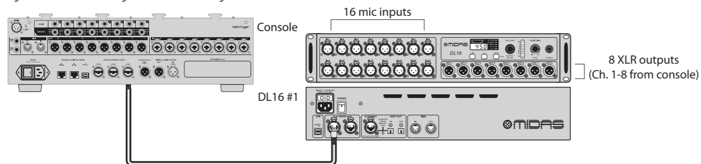
Fig. 1: Enkel enhetsinställning med DL16 i Standardläge
