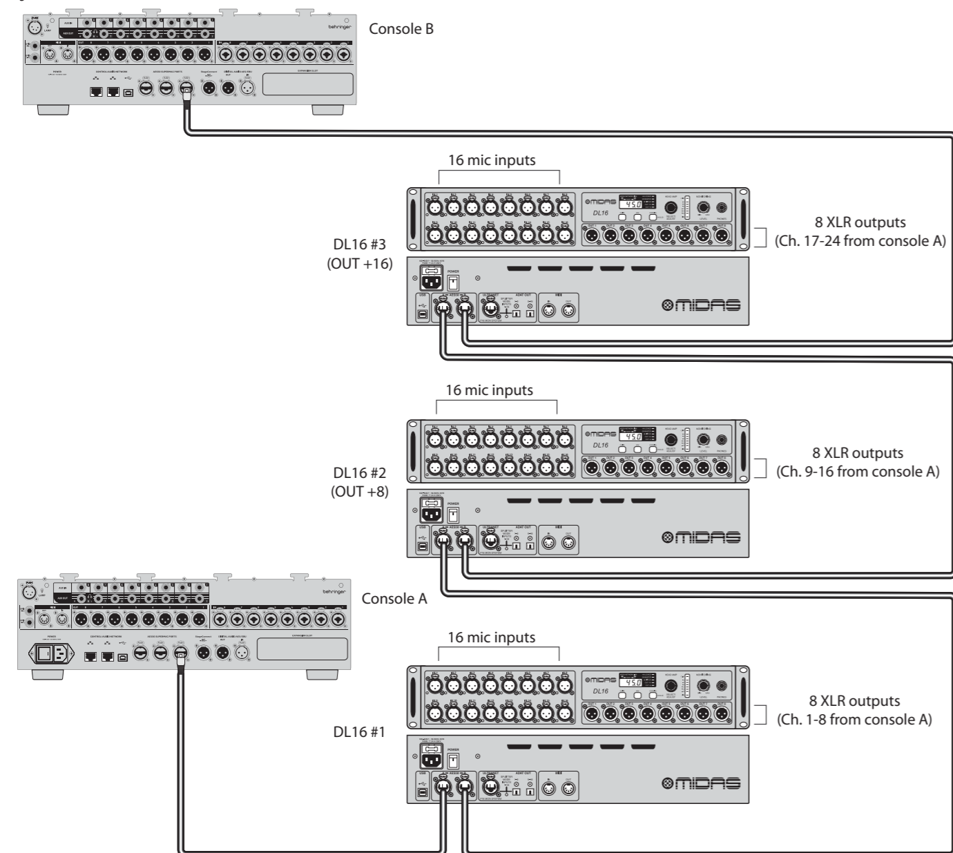
Fig. 3: Standard モード, Standard +8, および Standard +16 の DL16 での 3 ユニットのセットアップと2つのコンソール
