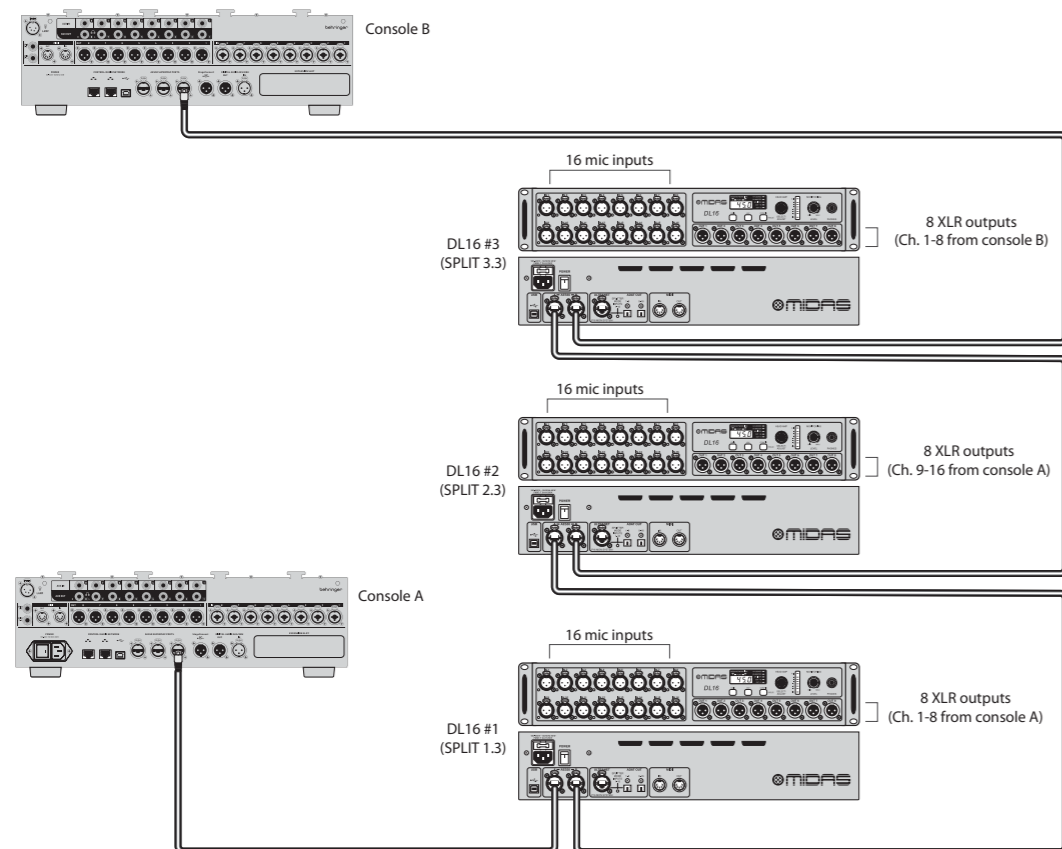
Fig. 4: Opstelling met drie eenheden met twee consoles en DL16's in Split 1.3, Split 2.3 en Split 3.3 modi
