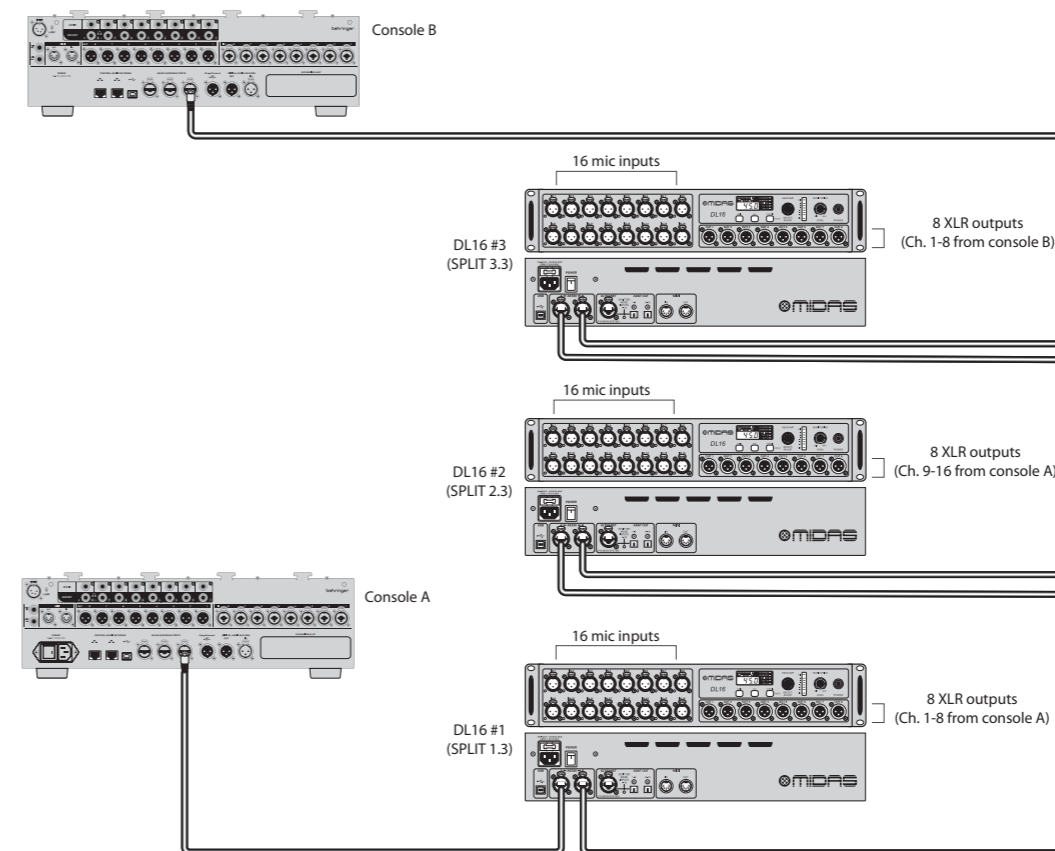
Abb. 4: Verwenden Sie das gleiche Setup wie oben gezeigt, konfigurieren Sie das erste DL16 im Split 1.3-Modus, Split 2.3 und Split 3.3-Modus.
