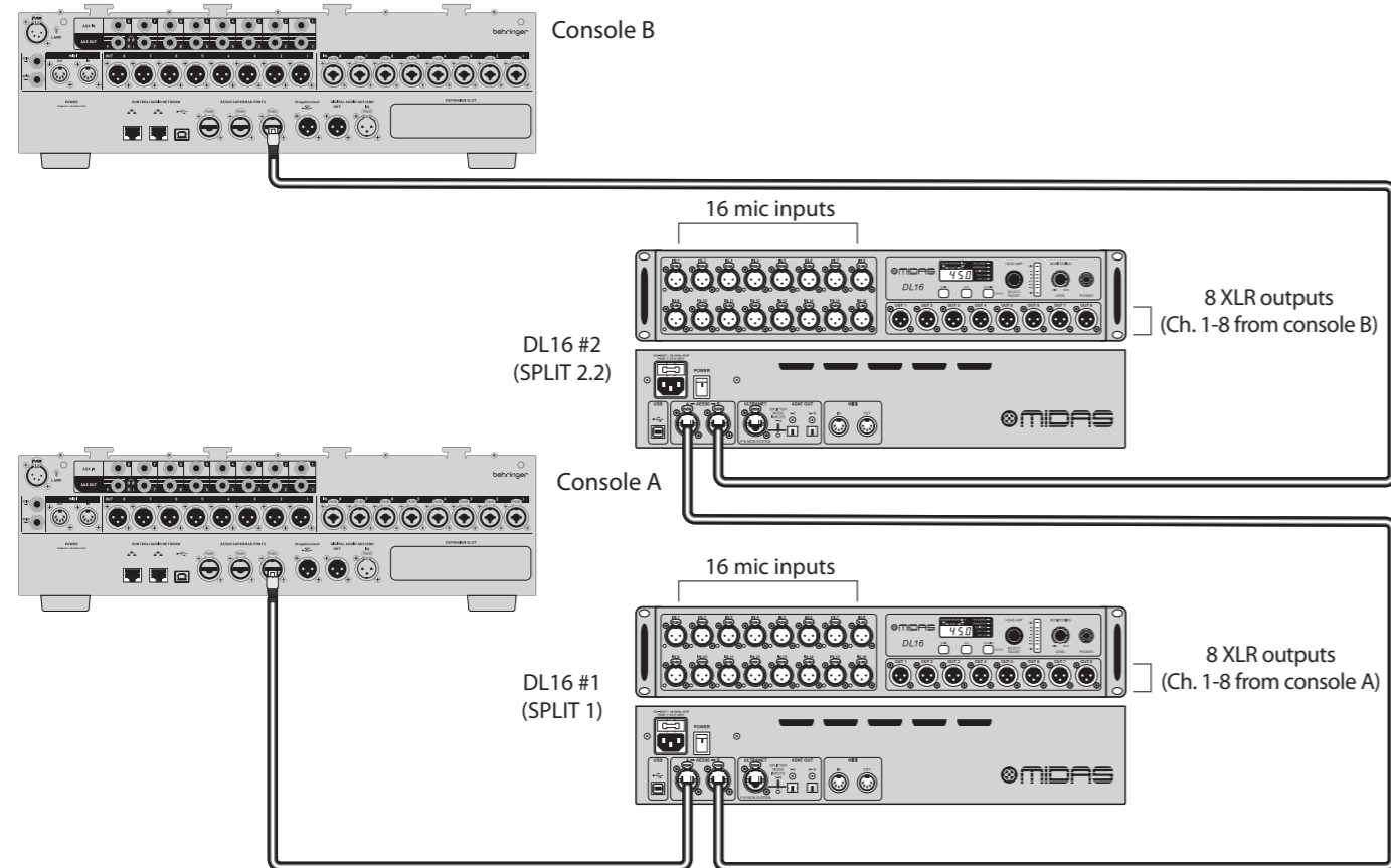
Fig. 5: Configuración de dos unidades con dos consolas y DL16s en modos Split 1.3 y Split 2.2
