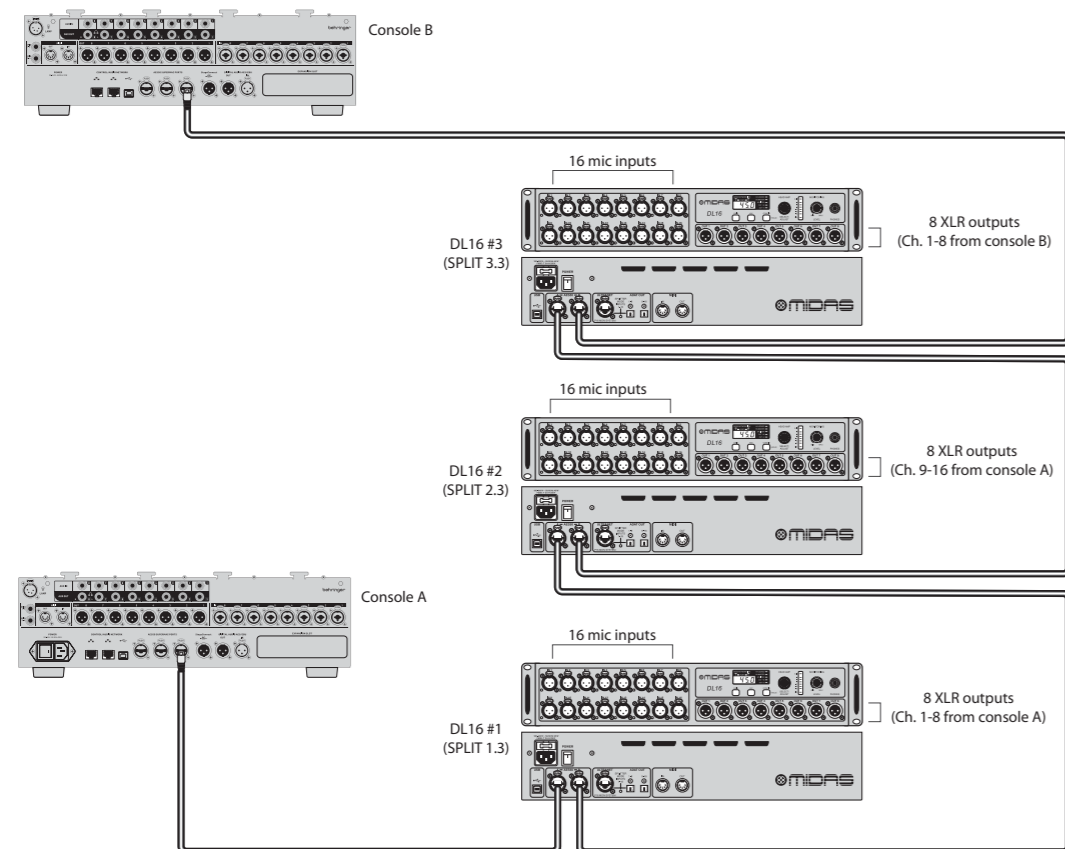
Fig. 4: Configuration à trois unités avec deux consoles et DL16s en modes Split 1.3, Split 2.3 et Split 3.3
