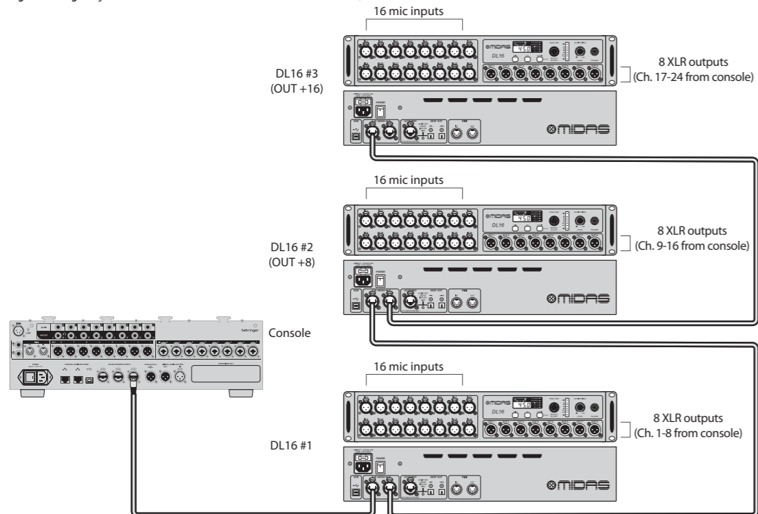
Fig. 2: Configuração de três unidades com DL16s no modo Padrão, Padrão +8 e Padrão +16
