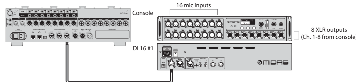
Rys. 1: Konfiguracja pojedynczej jednostki z DL16 w trybie Standard
