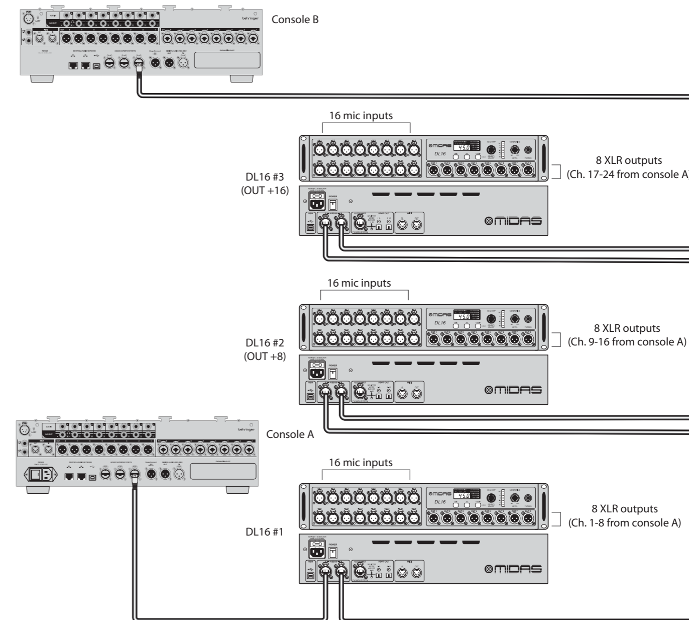
Fig. 3: Configuration de trois unités avec deux consoles et DL16 en mode Standard, Standard +8 et Standard +16
