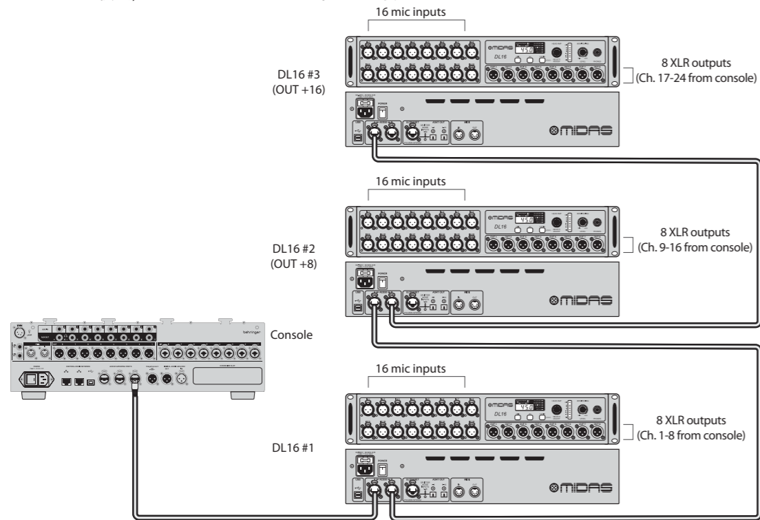
图 2: Standard 模式, Standard +8 和 Standard +16 的 DL16 三单元设置
