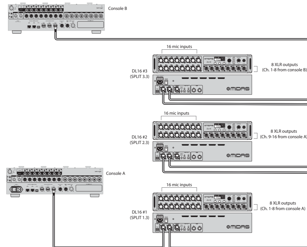
Fig. 4: Configurazione a tre unità con due console e DL16 in modalità Split 1.3, Split 2.3 e Split 3.3
