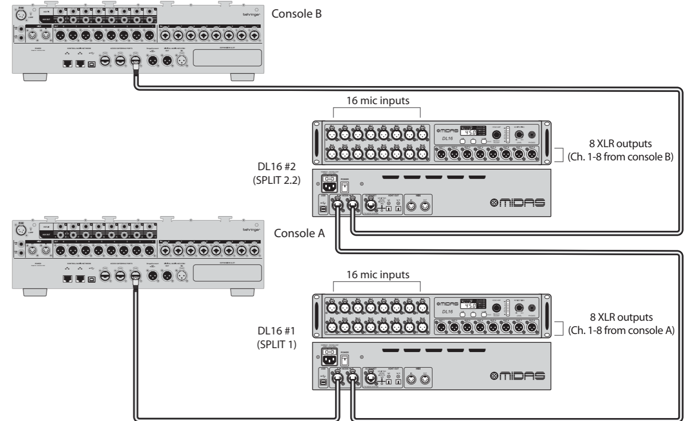
Rys. 5: Ustawienie dwóch jednostek z dwoma konsolami i DL16 w trybach Split 1.3 i Split 2.2
