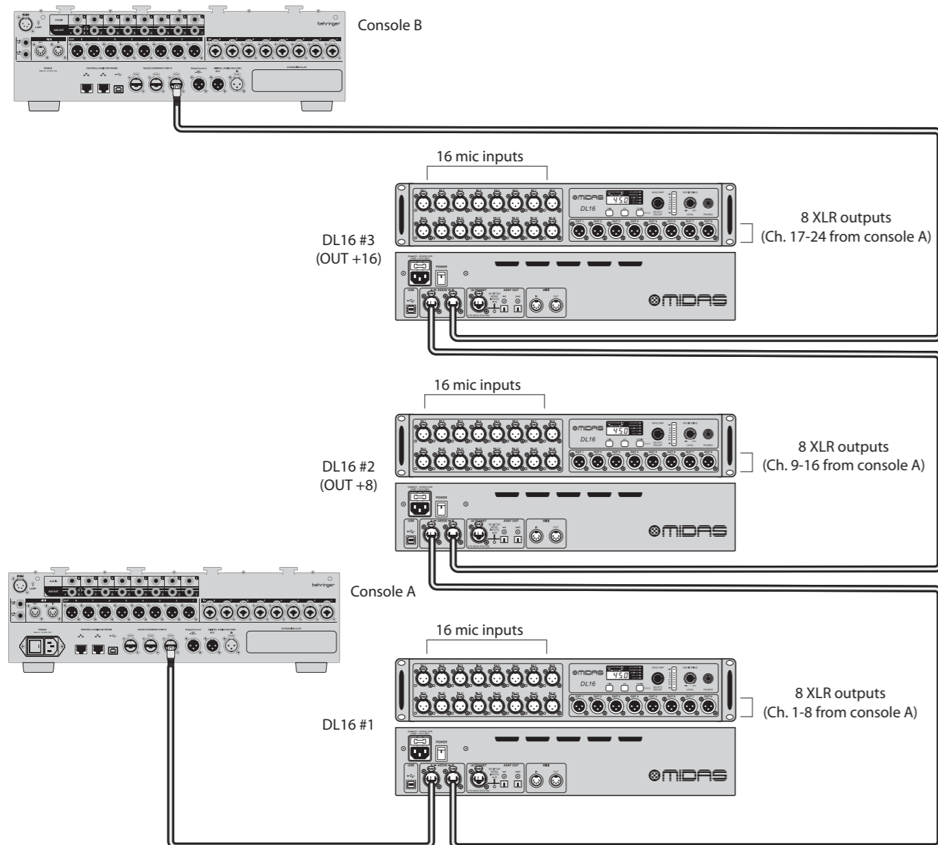
Fig. 3: Configurazione a tre unità con due console e DL16 in modalità Standard, Standard +8 e Standard +16
