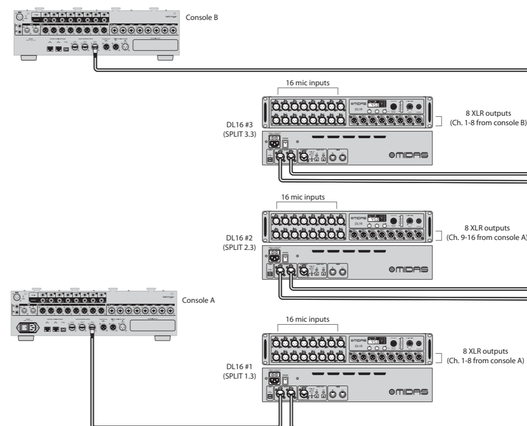
Fig. 4: Split 1.3, Split 2.3, および Split 3.3 モードの DL16 での 3 ユニットのセットアップと 2 つのコンソール
