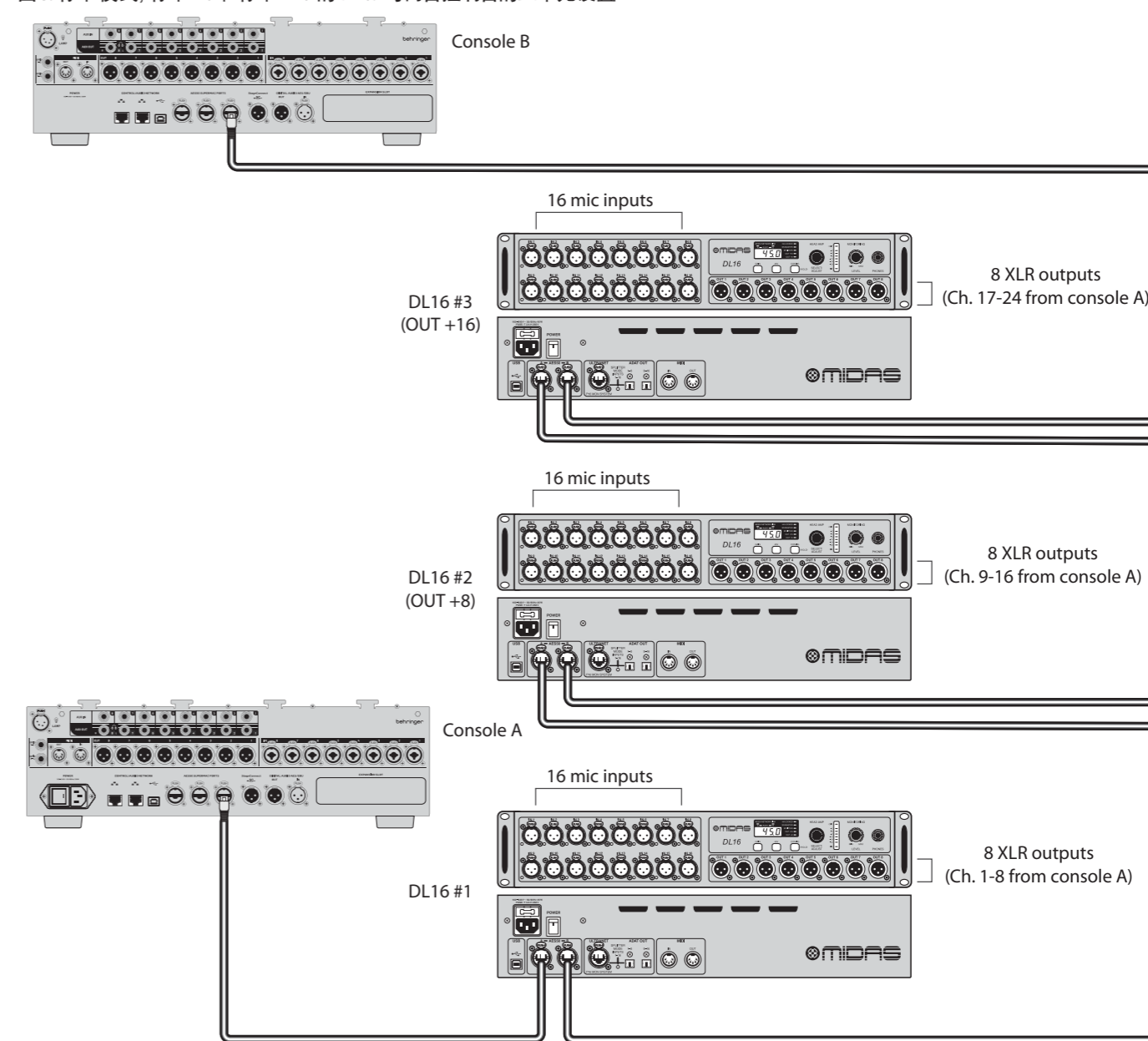
图 3: 标准模式, 标准 +8 和标准 +16 的 DL16s 与两台控制台的三单元设置
