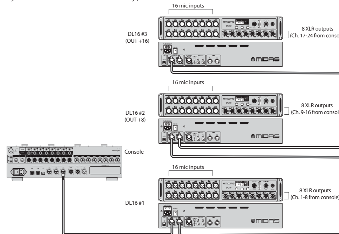
Fig. 2: Treenhetsinstallation med DL16 i Standardläge, Standard +8 och Standard +16
