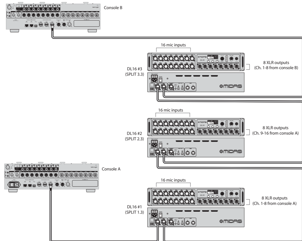
Fig. 4: Configuração de três unidades com duas consolas e DL16s nos modos Split 1.3, Split 2.3 e Split 3.3
