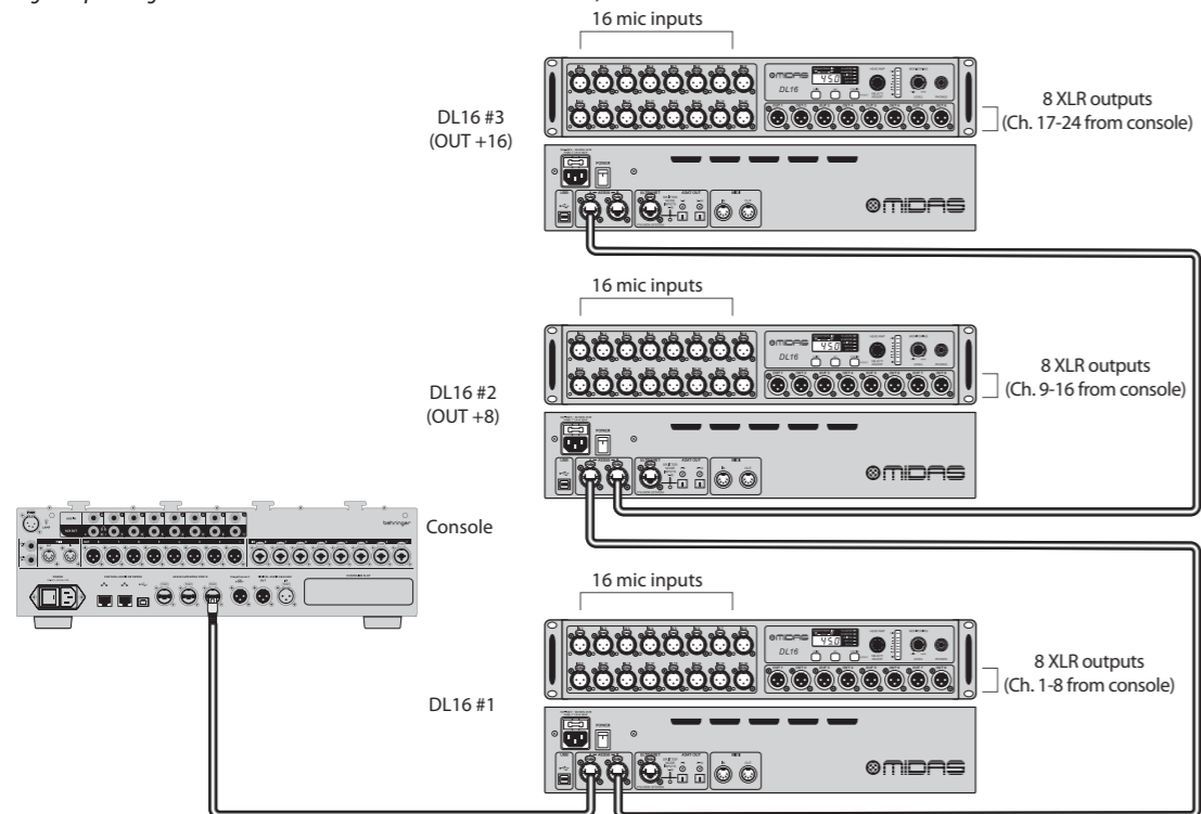
Fig. 2: Opstelling met drie eenheden met DL16's in Standaard modus, Standaard +8 en Standaard +16
