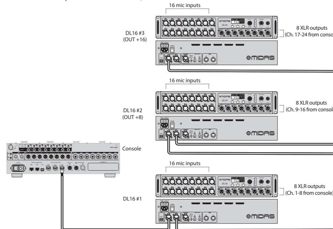
Abb. 2: Drei-Geräte-Setup mit DL16s im Standardmodus, Standard +8 und Standard +16
