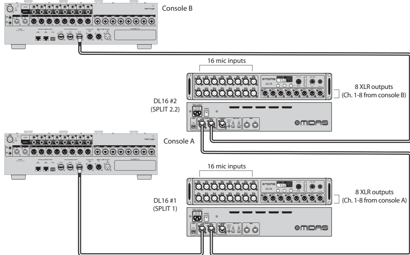
Fig. 5: Split 1.3 および Split 2.2 モードの DL16 を持つ 2 つのコンソールと 2 ユニットのセットアップ
