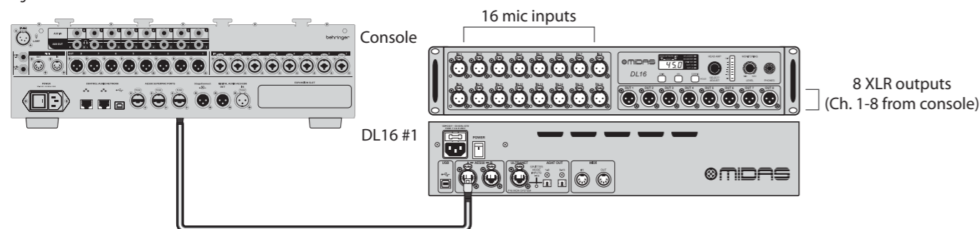
Fig. 1: Standard モードの DL16 での単一ユニットのセットアップ
