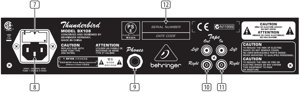
Kuva 1.2: Taustapuolen liitännät
