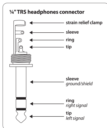
Fig. 4.2: Cablagem da ficha de jaque estéreo dos auscultadores e da ficha de jaque estéreo para o CD INPUT
