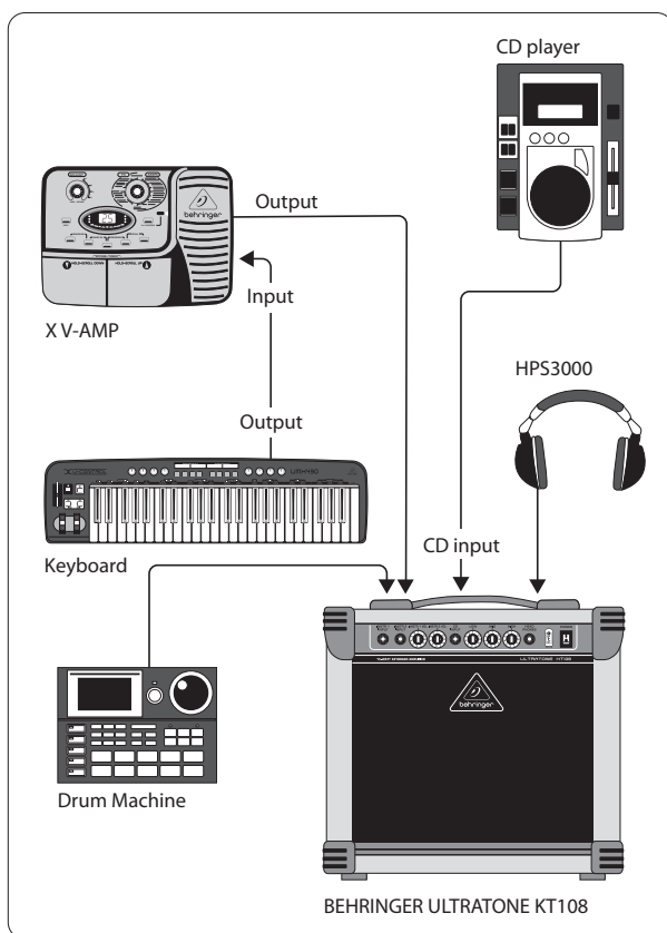
Fig. 2.1: Exemplo de montagem com o ULTRATONE KT108
