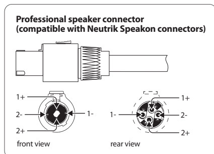
Εικ. 4.2: Επαγγελματική σύνδεση ηχείων με πόλωση
