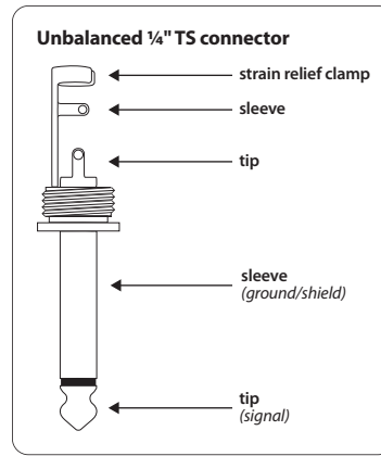
Kuva 4.3: 6,3 mm -monopistoke
