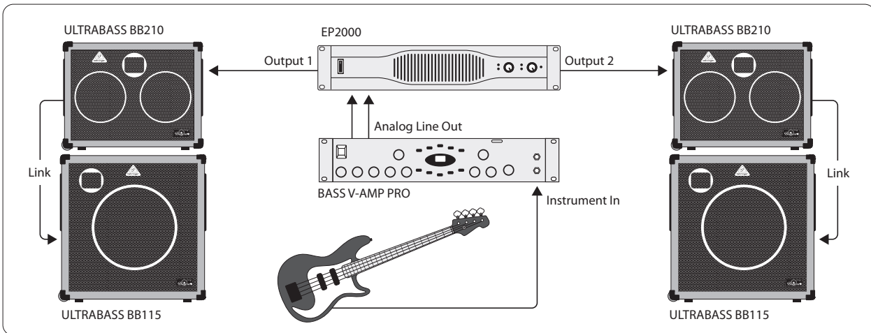
Kuva 3.4: Laajennettu stereo-kokoonpano
