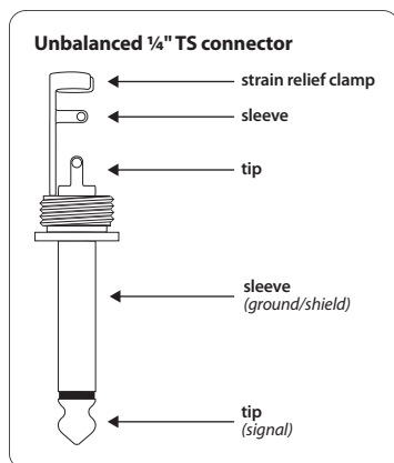
Afb. 3.2: 6,3 mm monoklinkerstekker
