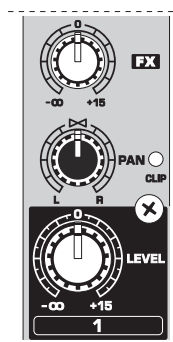
Afb. 2.3: De FX Send/panorama/level-regelaars
