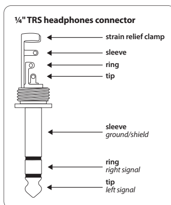
Afb. 3.4: Koptelefoon-stereoklinkerstekker
