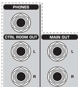
Afb. 2.9: Monitor-/Main Mix-aansluitingen
